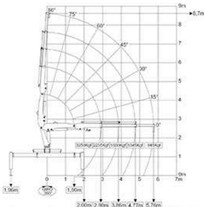
DIAGRAMA OPERACIONAL DE CARGAS Y ALCANCES GRUA VEHICULAR CA6.5-5,7/21
