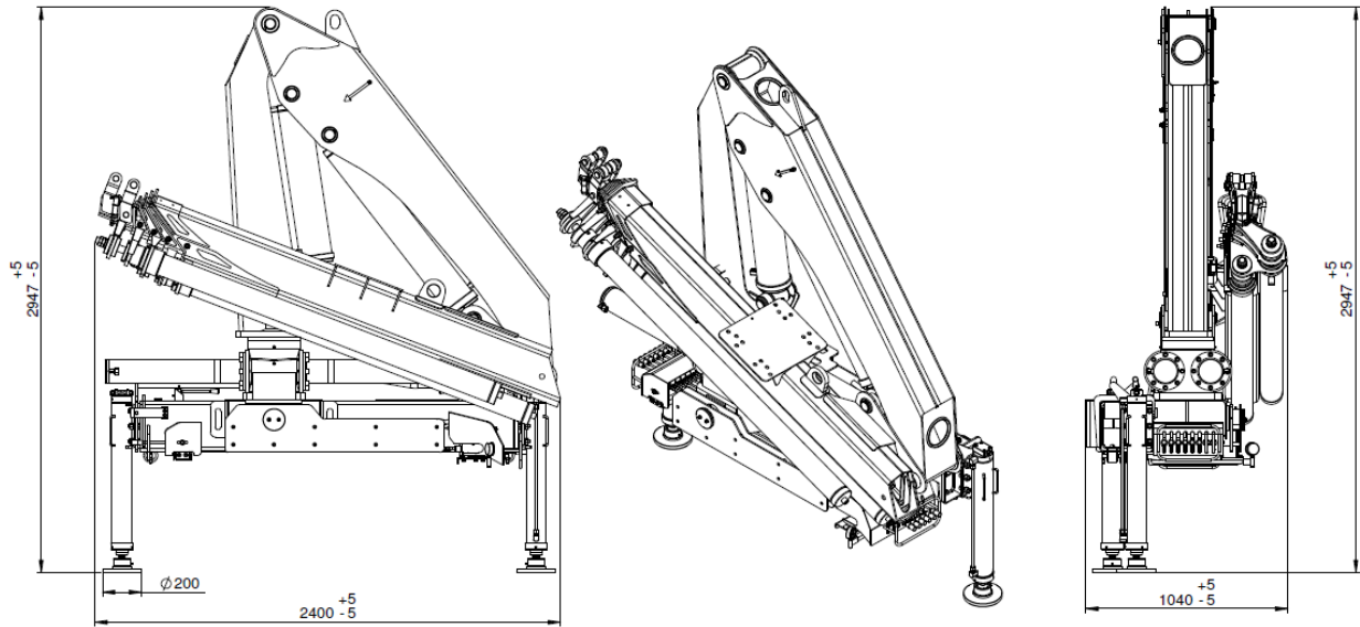
Dimensiones aproximadas
